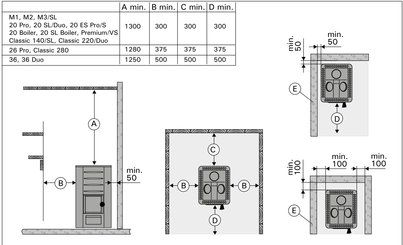
Рисунок 7. Безопасные расстояния (все размеры приведены в миллиметрах) Joonis 7. Ohutuskauused (kõik mõõtmised millimeetrites)
